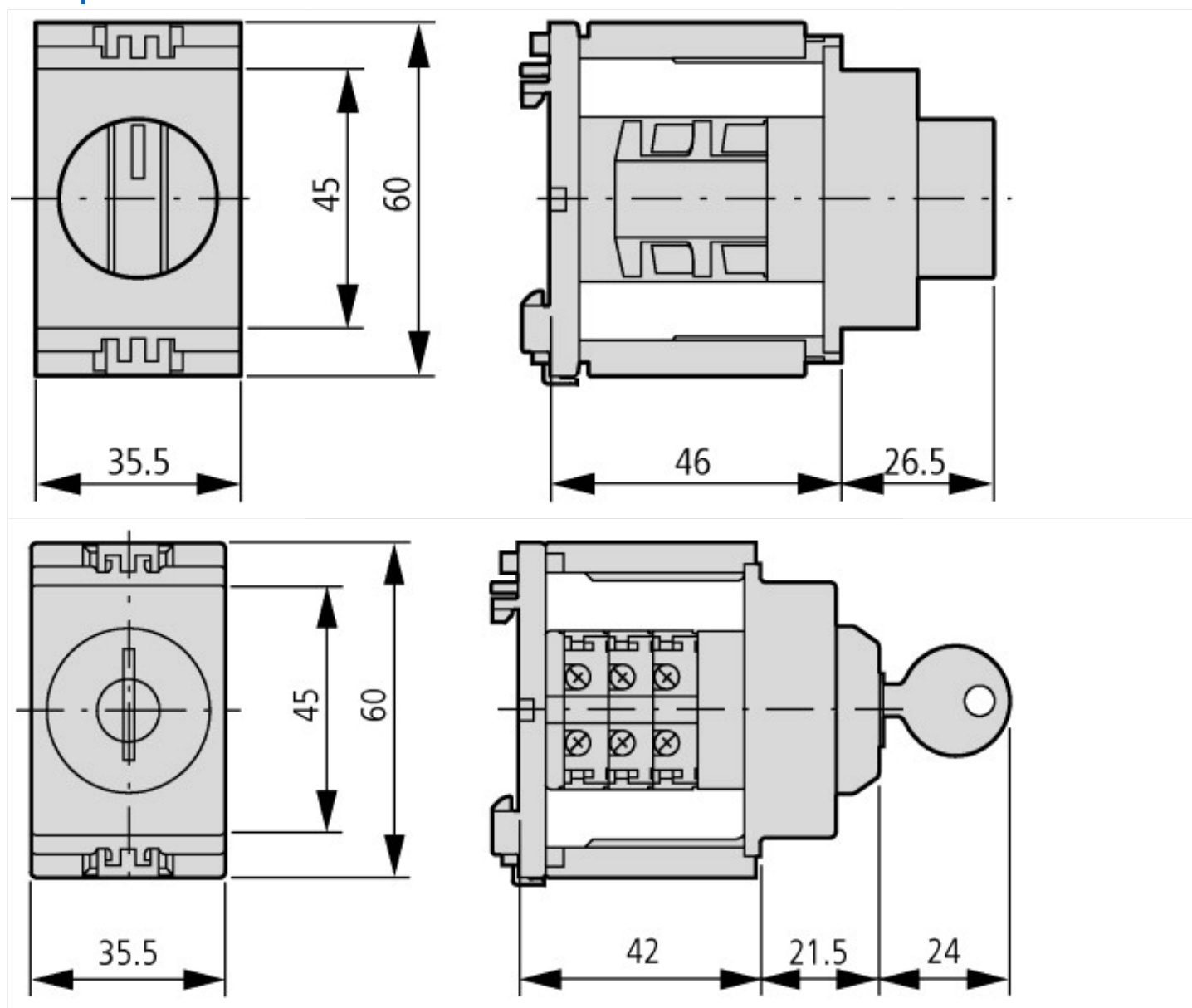
Механизм блокировки работы с ключом
