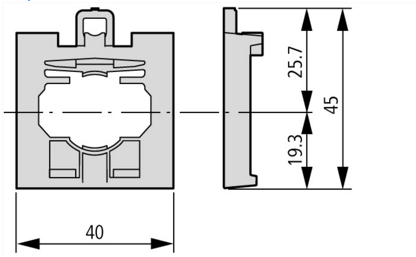
Крепёжный адаптер Крепежный адаптер (фронтальная установка) для 3 контактных/светодиодных индикаторов
