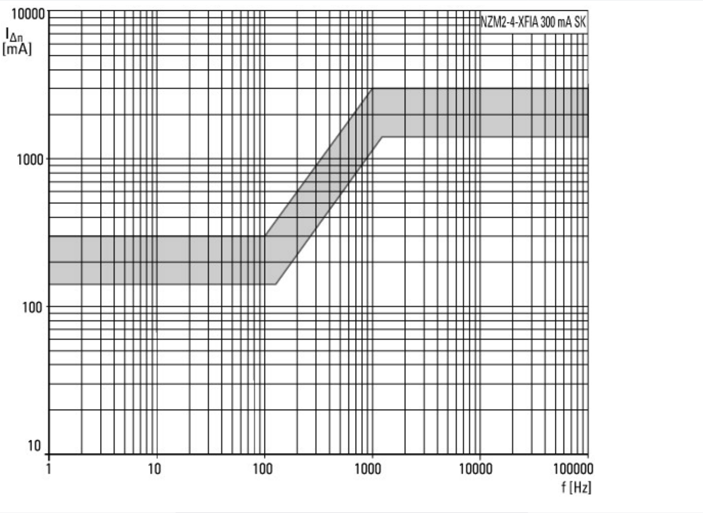
Зависимость от частоты тока расцепления 300 mA Тип SK
