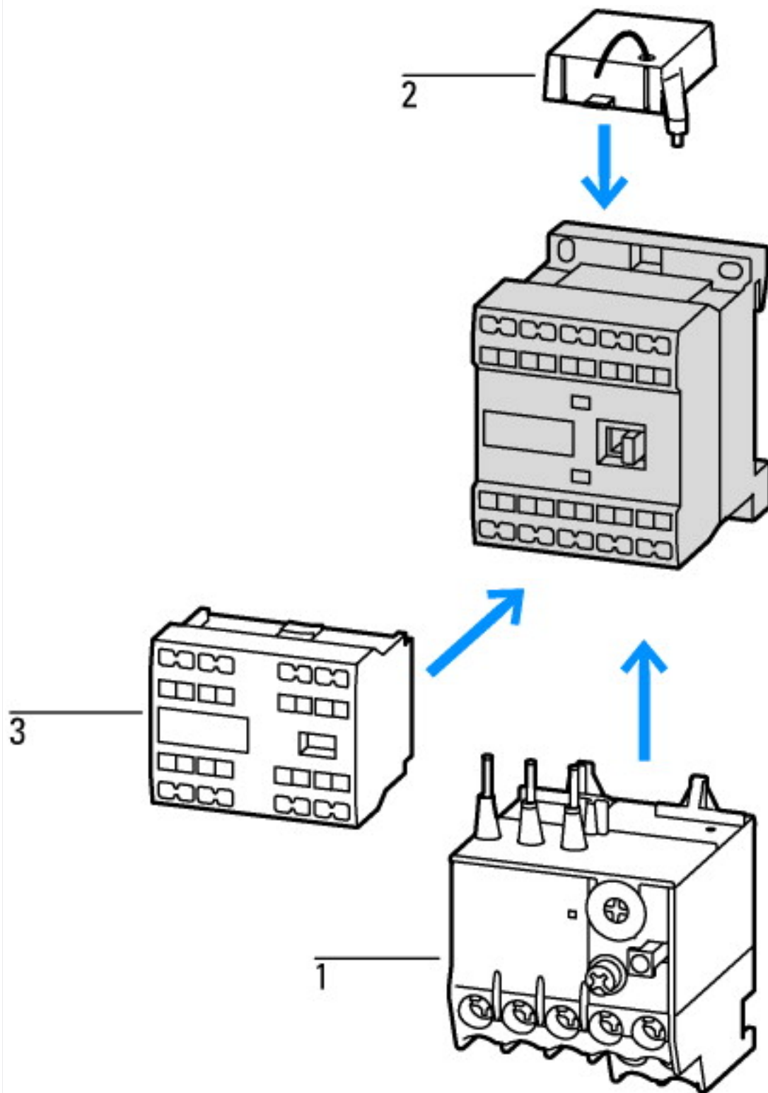
1: Реле защиты электродвигателей 2: Схема защиты 3: Модули вспомогательных контактов Корпус полностью изолирован
