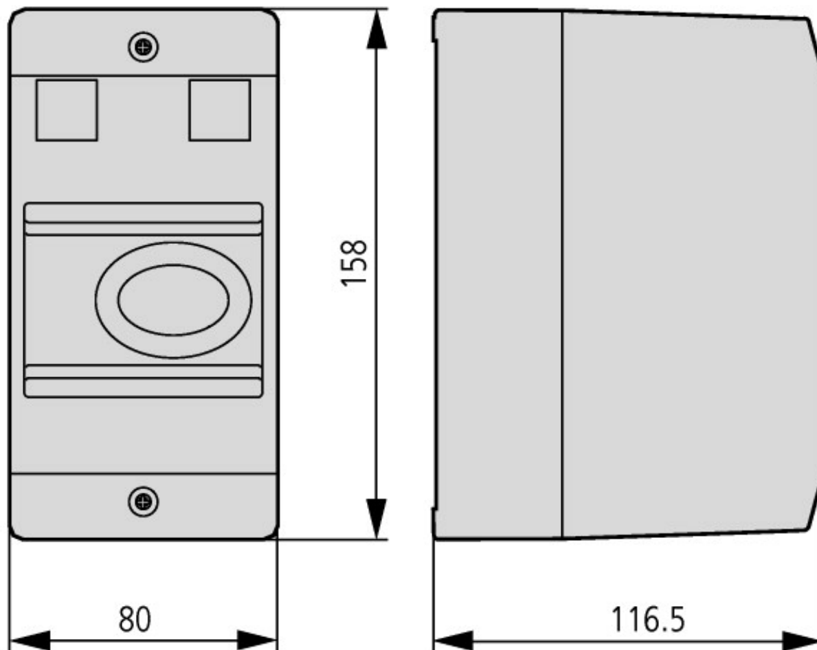
Изолированный корпус для монтажа на поверхность
