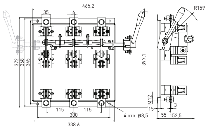
Рис. 4 - Габаритные и установочные размеры разъединителя типа РПБ-630
