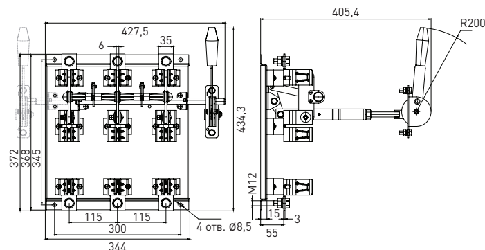
Рис. 8 - Габаритные и установочные размеры разъединителя типа РПС-630
