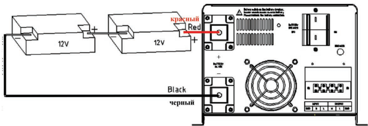
Схема подключения аккумуляторных батарей U=24B . Модель PSW-HW 2500–3500 Вт
