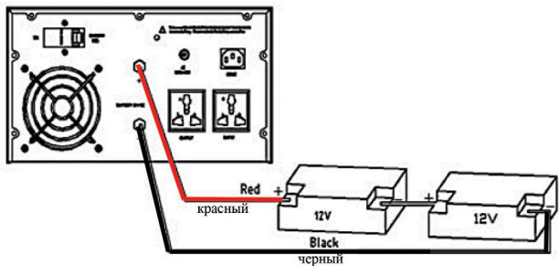
Схема подключения аккумуляторных батарей U=24B . Модель PSW-H 1600 Вт
