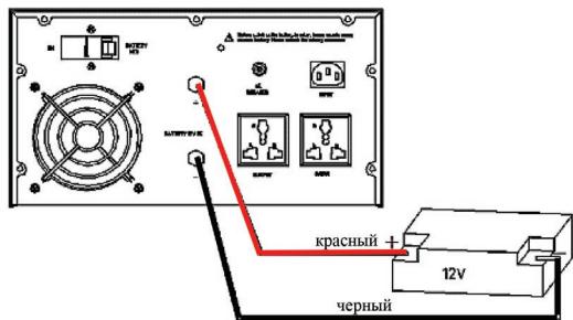
Схема подключения аккумуляторных батарей U=12B . Модель PSW-H 300–1000 Вт
