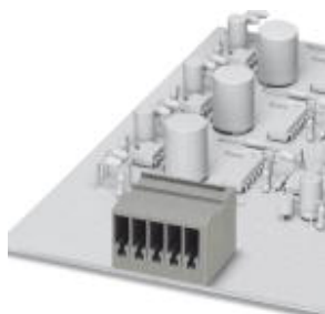
Устройство сопряжения ST-COMBI, подключение параллельно печатной плате, шаг: 5,2 мм, количество контактов: 10
