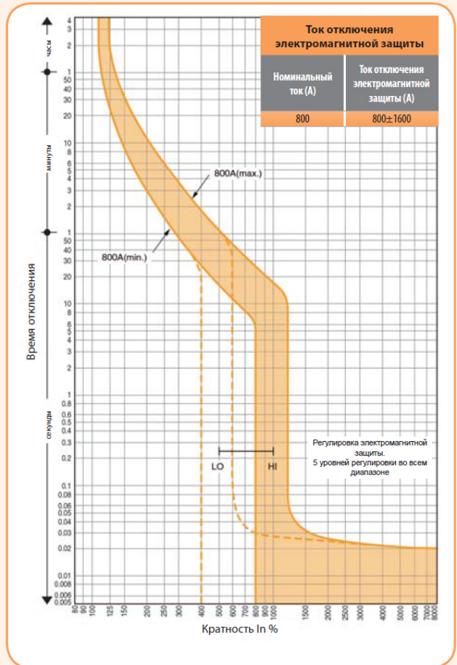
EB2 800 (800A) Характеристика t-I
