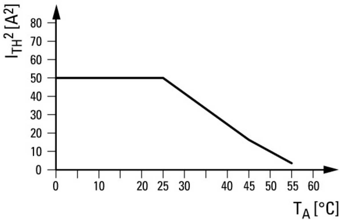
Кривая дерейтинга
