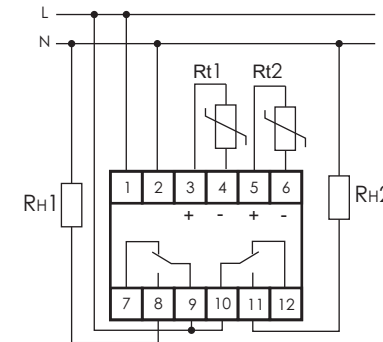
Схема подключения при нагрузке до 16А.
